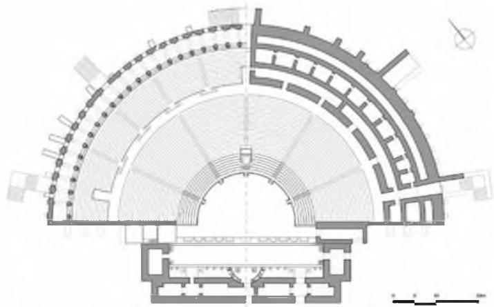
Θέατρο. Κάτοψη της δεύτερης οικοδομικής φάσης
