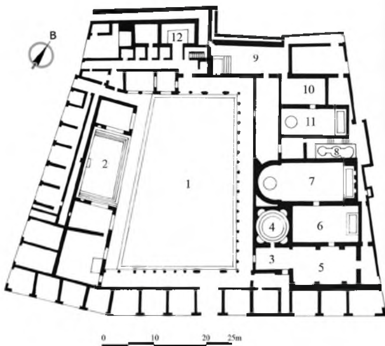
Σταβιανές Θέρμες της Πομπηίας, κάτοψη
