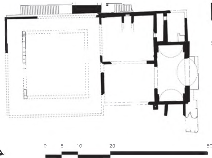
Κάτοψη του Βαλανείου, νότια του Ωδείου
