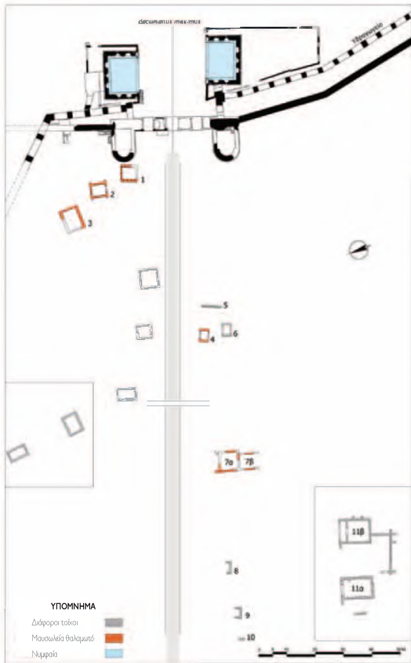
Κάτοψη της Δυτικής Νεκρόπολης
