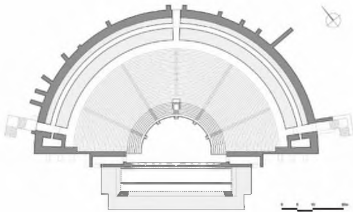
Θέατρο. Κάτοψη της πρώτης οικοδομικής φάσης
