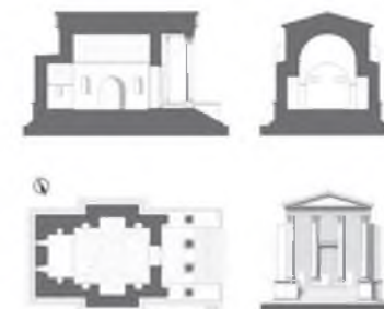
Το ναόσχημο Μαυσωλείο 2 και η γραφική του αναπαράσταση
