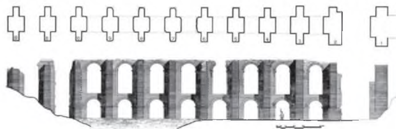
Κάτοψη και όψη της νότιας πεσσοστοιχίας (γέφυρας) στις πηγές του Αγίου Γεωργίου
