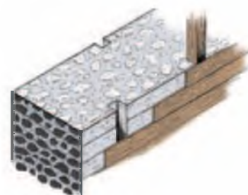
I. Opus caementicium
