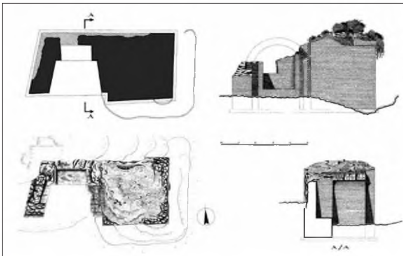
Κάτοψη και όψεις του Υδατόπυργου
