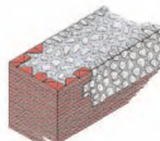
VI. Opus mixtum
