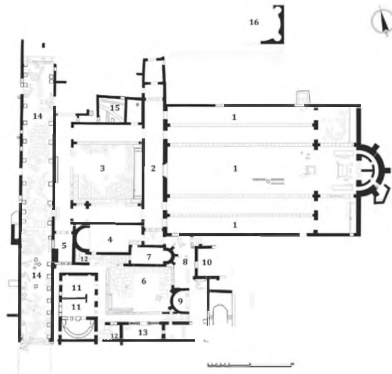
Κάτοψη της Βασιλικής Β
