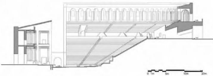
Θέατρο. Τομή της δεύτερης οικοδομικής φάσης
